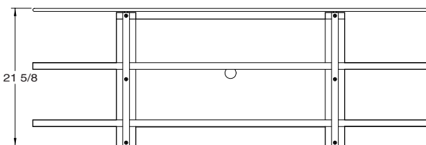
DIAZ BTV 1862 02 VUE DE FACE / FRONT VIEW
